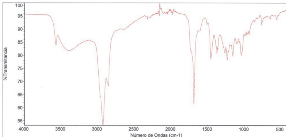
Fig. 3. Espectro infrarrojo del componente ACF
