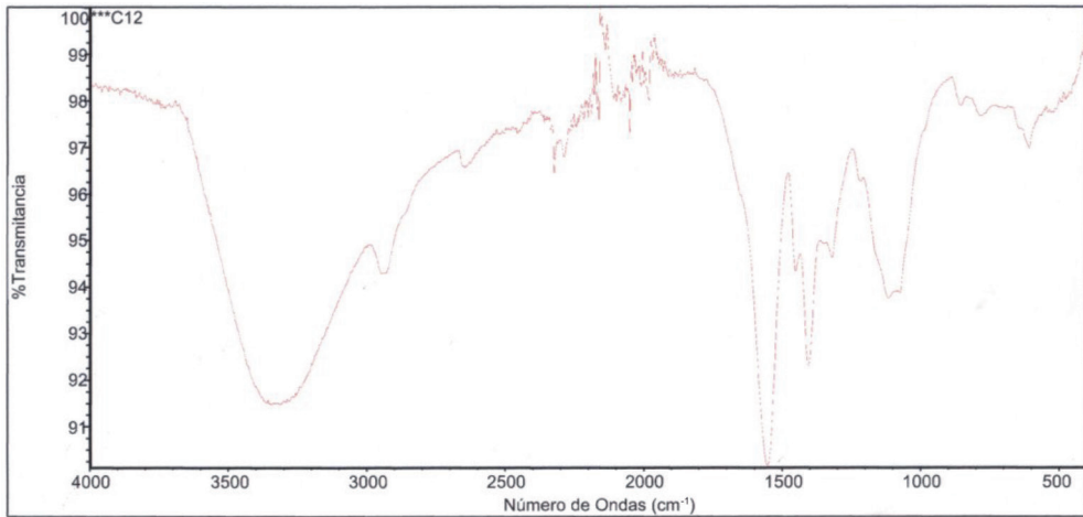
Fig. 1. Espectro infrarrojo del componente C12AAg
