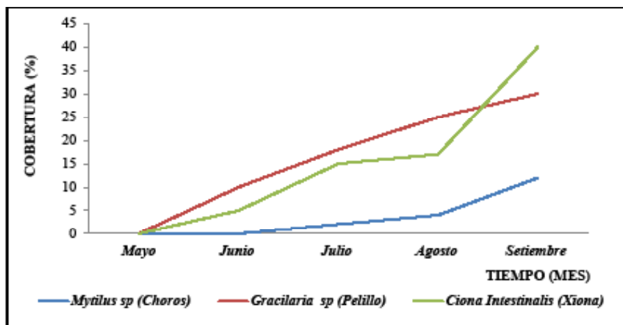
Fig. 3. Evolución de la cobertura del fouling en la estación B (Sin antifoulig) de la Bahía de Guaynuná, 2014.
