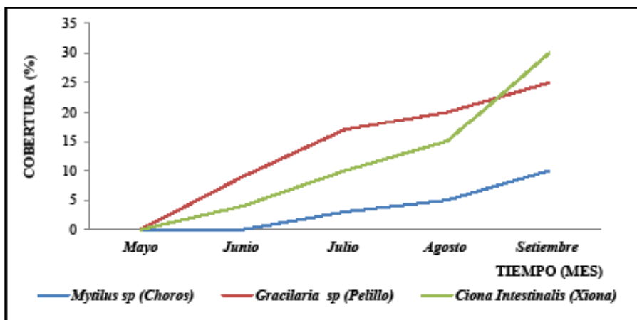
Fig. 4. Evolución de la cobertura del fouling en la estación A (Con antifouling) de la Bahía de Guaynuná, 2014.
