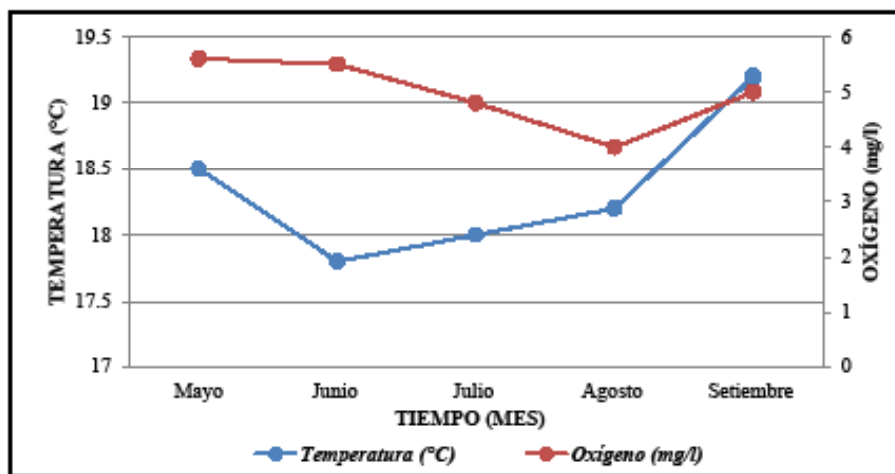
Fig. 2. Variación de la temperatura y el oxígeno de la Bahía de Guaynuná.
