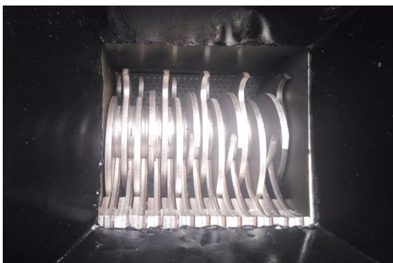
Figura 5. Vista real hacia el interior de la tolva que contiene a la herramienta para triturar PET.
