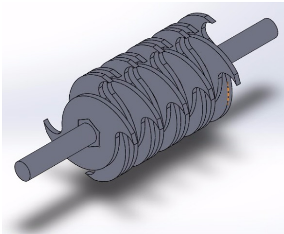
Figura 2. Simulación mediante Solidworks de la herramienta a usar por el prototipo para triturar PET.
