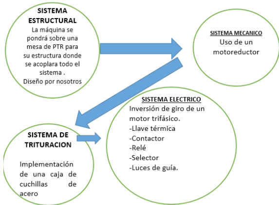
Figura 8. Lógica de implementación de la máquina trituradora de PET desarrollada en el proyecto.
