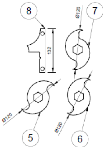
Figura 1. Dimensiones de las cuchillas a usar para triturar plásticos PET.
