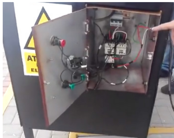
Figura 7. Caja eléctrica de mando de la máquina trituradora de PET
