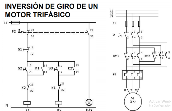
Figura 6. Lógica de inversión de giro del motor trifásico utilizada e implementada en el proyecto.
