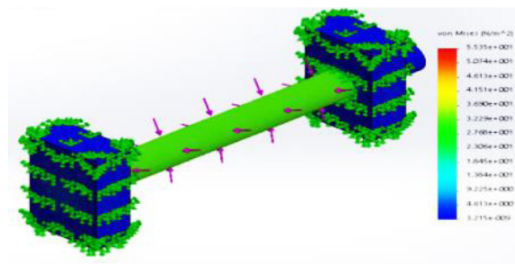
Figura 3. Fuerzas aplicadas al eje que contendrá a la herramienta trituradora de material PET.
