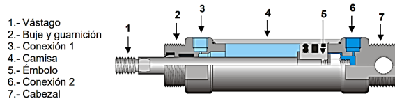
Figura. 7. Cilindro de doble efecto (Festo).
