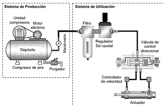
Figura. 6. Sistema electroneumatico usado en el proyecto (Festo)
