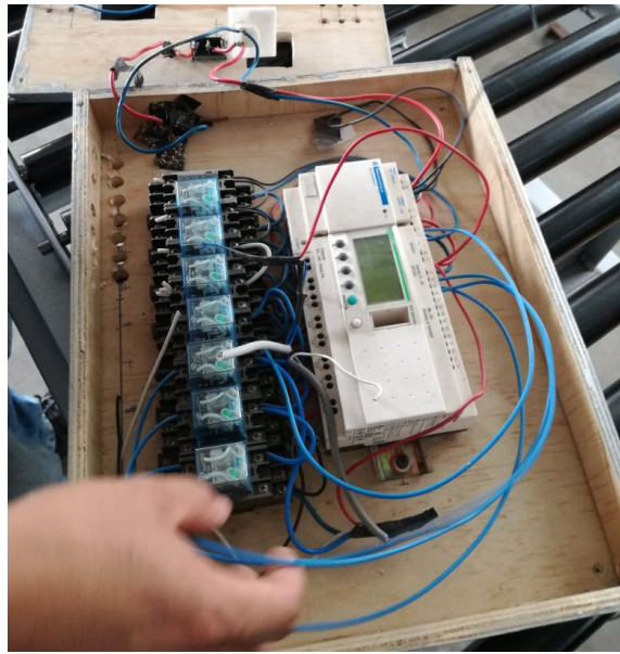
Figura. 8. PLC (caja blanca) y relés usados en el proyecto.
