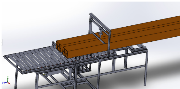
Figura. 3. Diseño en CAD del equipo desarrollado en este trabajo.
