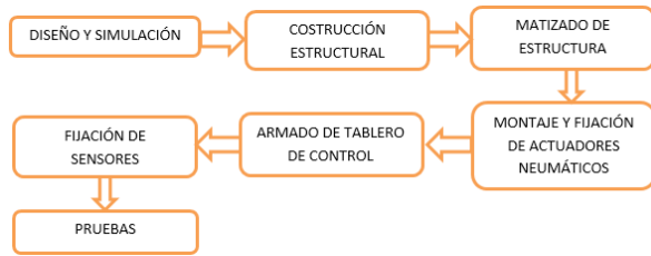
Figura. 1. Diagrama lógico fundamental de la implementación de la máquina de corte de arcilla.
