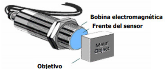
Figura. 8. Sensor inductivo usado en el proyecto (Festo).
