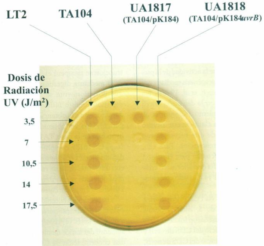
Figura 7. Placa mostrando la sensibilidad a la radiación UV de las construcciones UA1817 y UA1818
