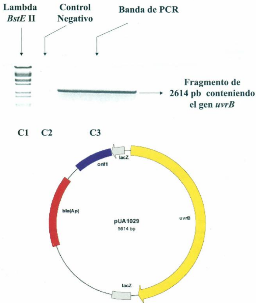
Figura 4. Electroforesis mostrando el fragmento de PCR conteniendo el gen uvrB de S. enterica Typhimurium LT2 y representación esquemática del plásmido pUA1029, producto de la ligación del fragmento conteniendo el gen uvrB en el vector pGEM ® -T
