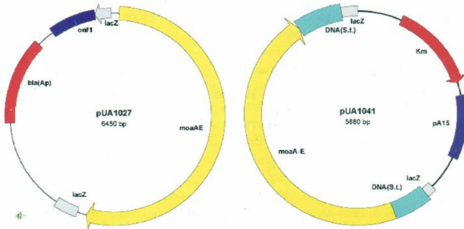
Figura 2. Esquema del plásmido pUA1027 (producto de la ligación del fragmento conteniendo el operón moa en el vector pGEM ® -T) y plásmido pUA1041 (producto de la ligación del fragmento conteniendo el operón moa en el vector pK184)
