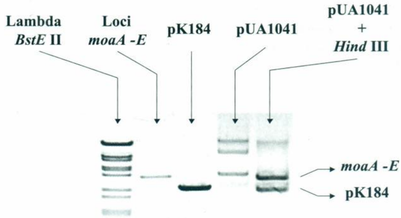
Figura 3. Electroforesis mostrando la liberación del operón moa del plásmido pK184, mediante digestión con Hind III del plásmido pUA1041
