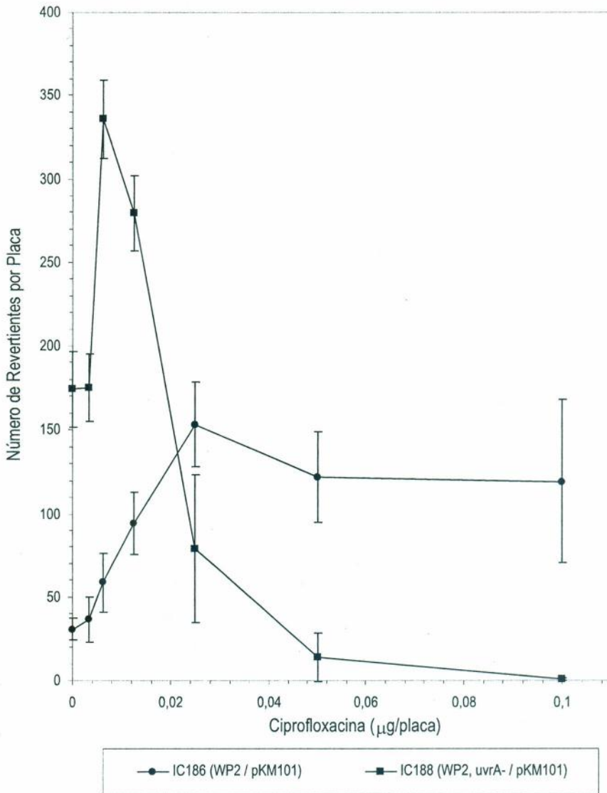
Figura 8. Número de revertientes por placa a diferentes dosis de ciprofloxacina, en cepas uvrA - y uvrA + de E. coli WP2
