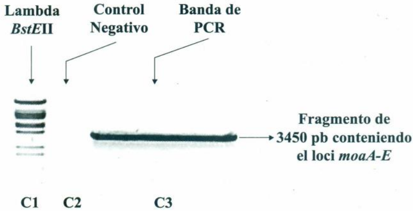
Figura 1. Electroforesis mostrando el fragmento de PCR conteniendo el operón moa de S. enterica Typhimurium Lt2
